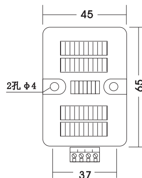
复合式传感器外形尺寸图
