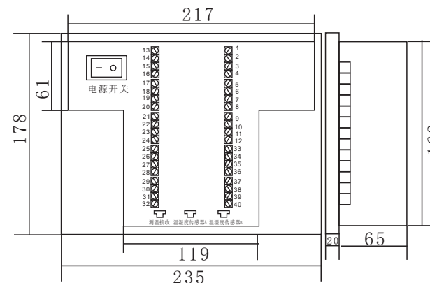
外形尺寸: 235×178×85
