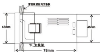
面板(嵌入)式安装 开孔尺寸为:45X45mm
