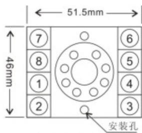
基座(导轨)安装座 置入35mm导轨中
