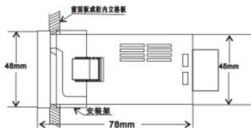
面板(嵌入)式安装 开孔尺寸为:45X45mm
